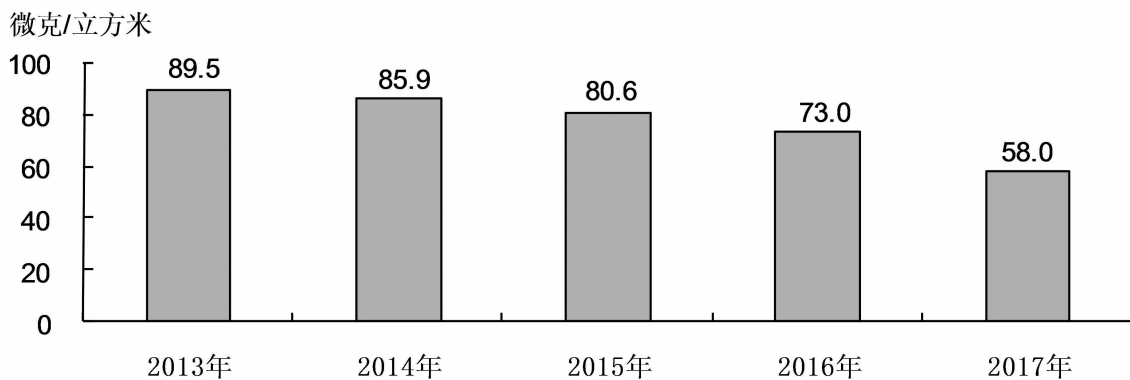
图 13 2013—2017 年细颗粒物(PM 2.5 )年均浓度
