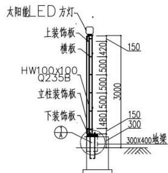
3m围挡剖面图
