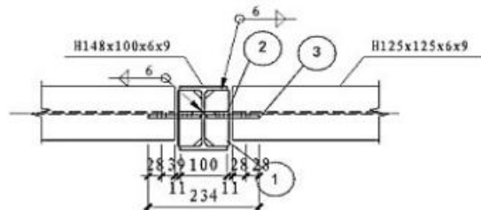
A2 2-2剖面图
