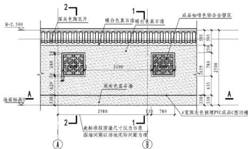
正立面图
