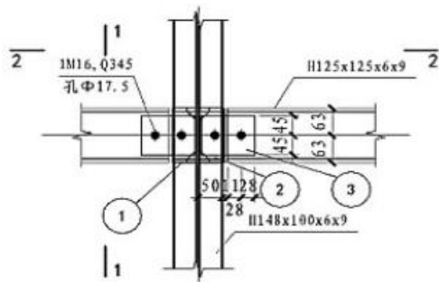
节点A2 侧视图
