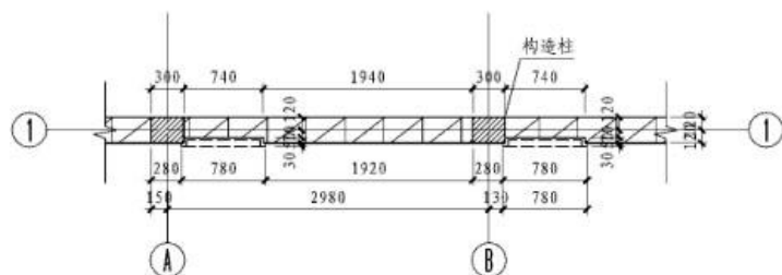
A-A断面图
