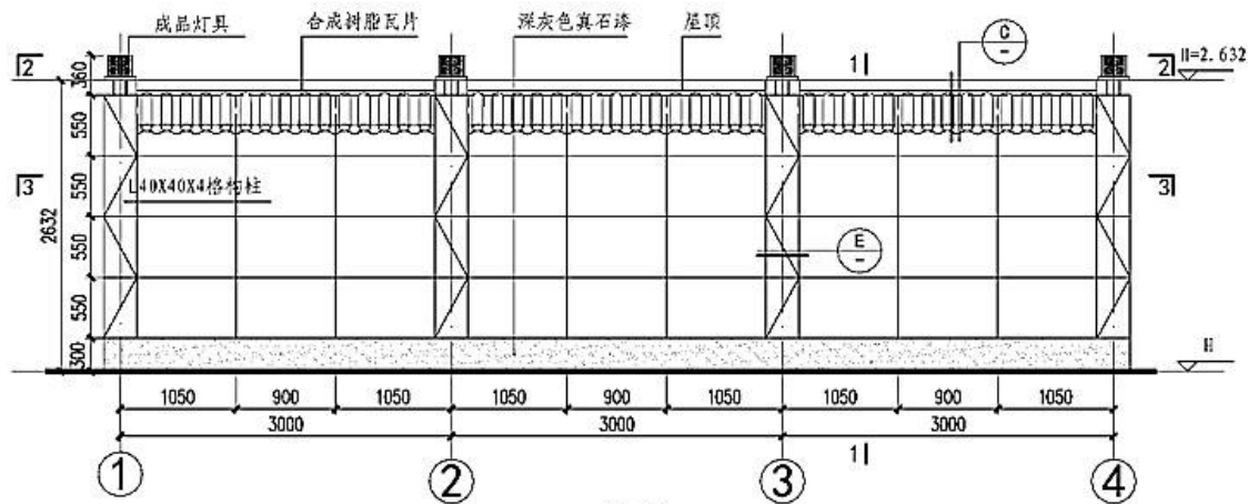
立面图
