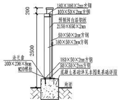
1-1剖面图
