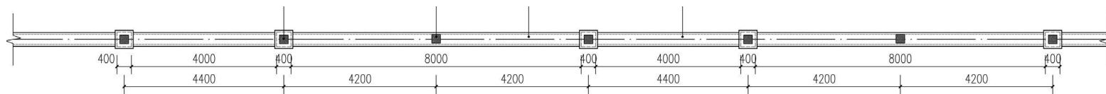
砌筑式围挡平面示意
