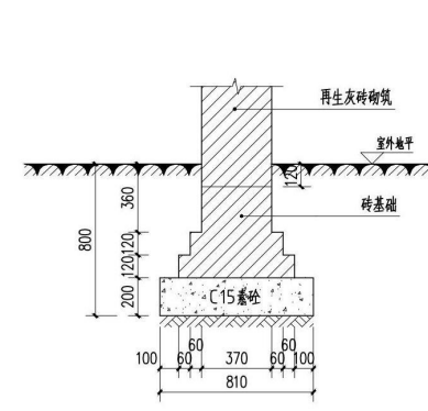
砖墙基础 1:20
