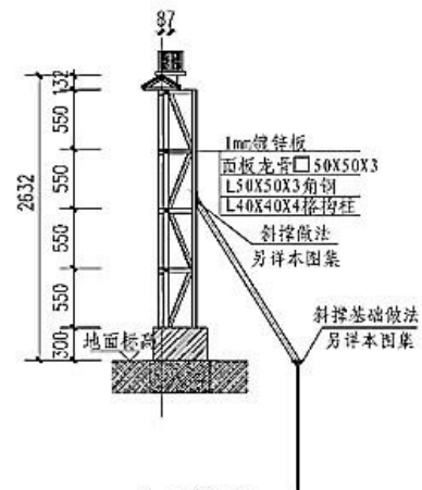
1-1剖面
