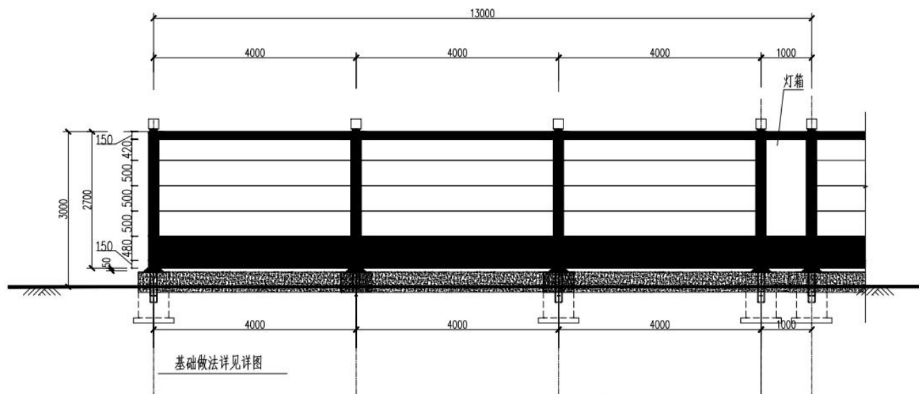
3m围挡立面图
