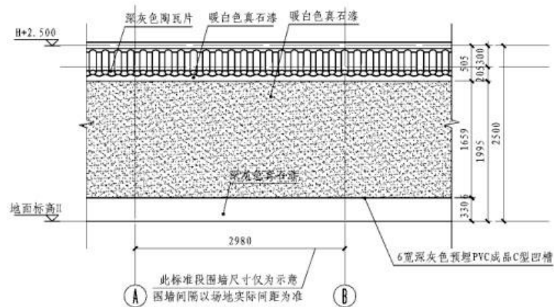
背立面图
