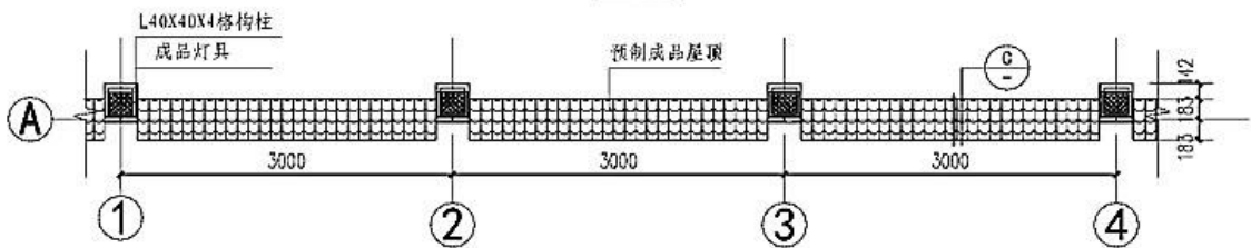
2-2顶视图
