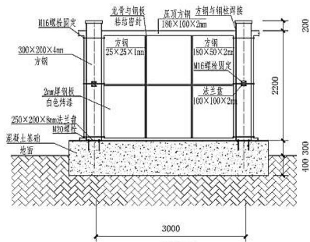
背视图
